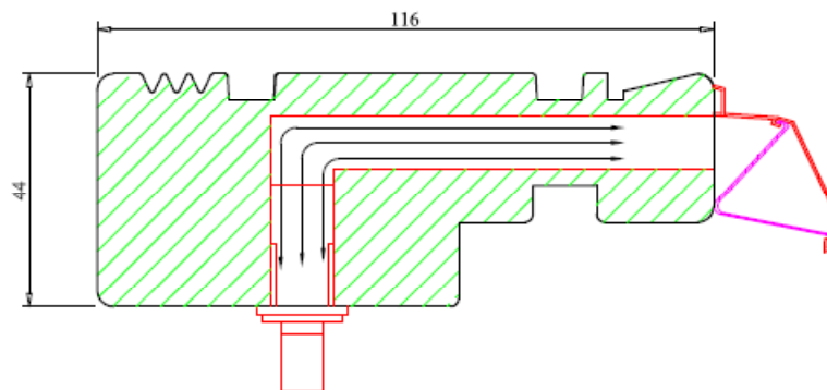
Synlig ventilation
